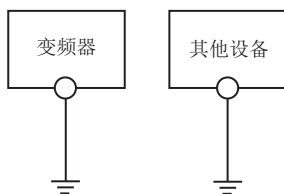
(I) 专用接地…最好
