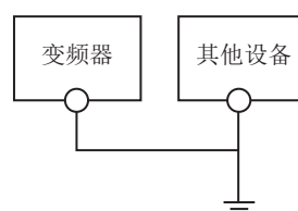
(III) 共通接地…不可
